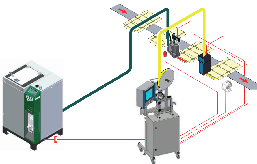
Heissleimauftrag mit Schmelzgerät JumboFlex oder Concept und Flächenauftragskopf FK IT
