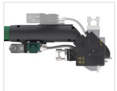
Magnetbleche oben und unten zur Befestigung des Magnetventils
