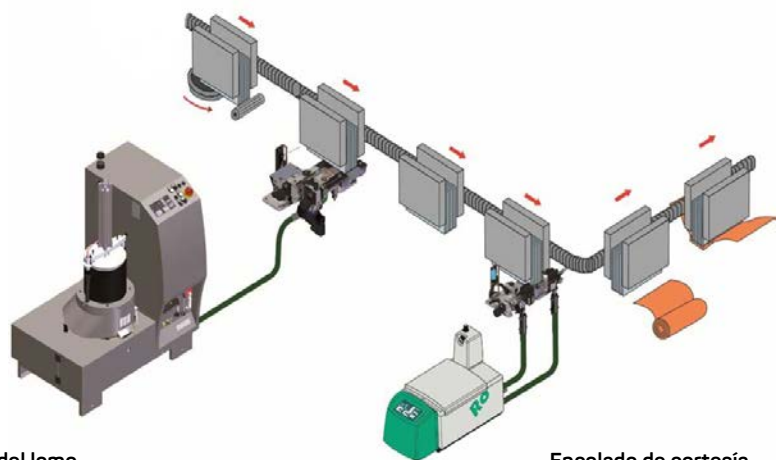
Encolado del lomo RobaPUR 35 MOD SpineCoat 65 o 80
