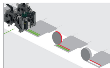
Aufreissfaden und Haftklebeverschluss parallel geklebt
