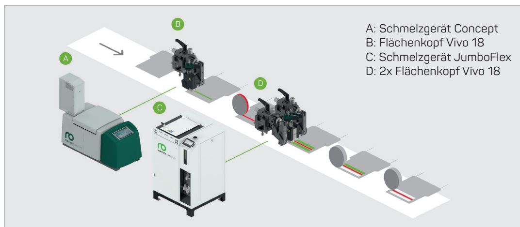
Aufreissfaden kombiniert mit Haftklebeverschlüssen
