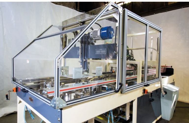
带有自动加料系统与 GlueFill 颗粒胶料桶 (右) 的托盘成型机
